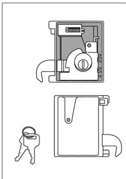
錠前セット (旧)
